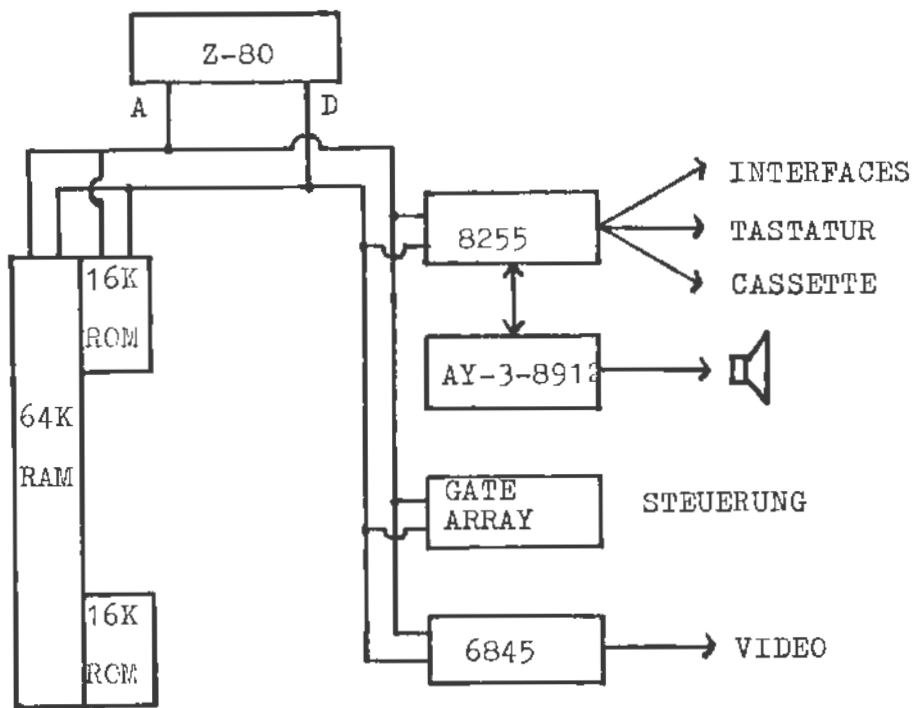
Abb. 1 Der Aufbau des CPC-464
